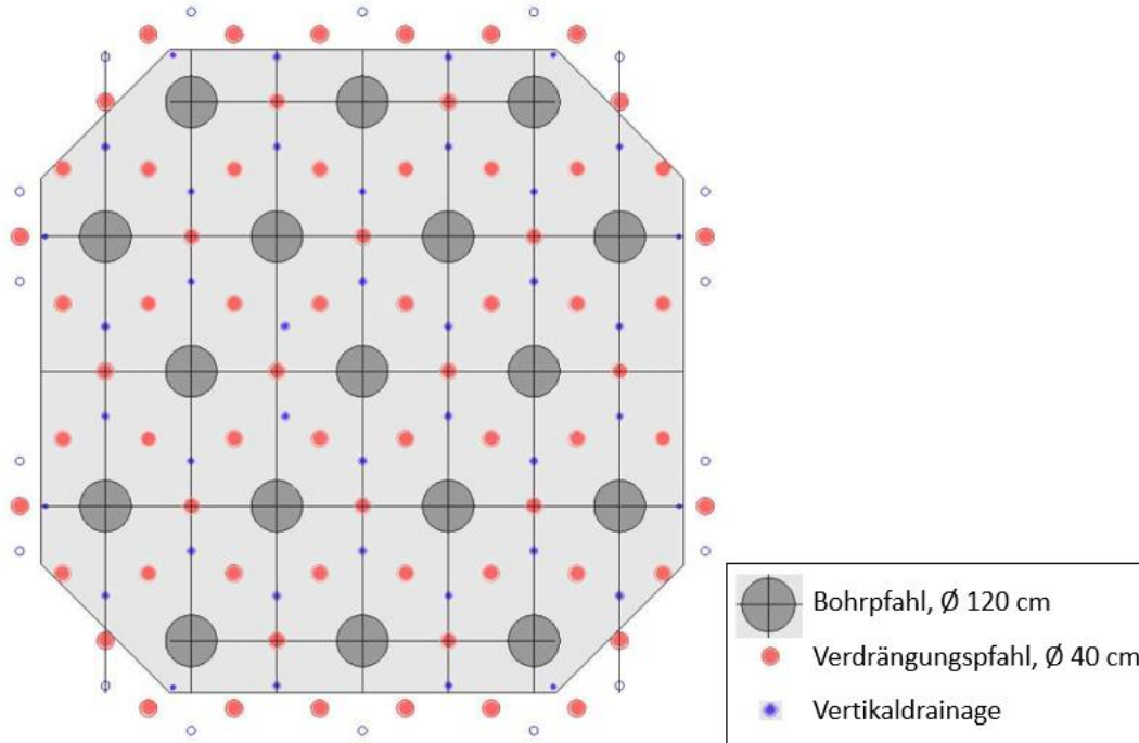
Schematische Grundung der Aicherparkbrücke unter den Pfeilerscheiben (Grafik: TUM)
